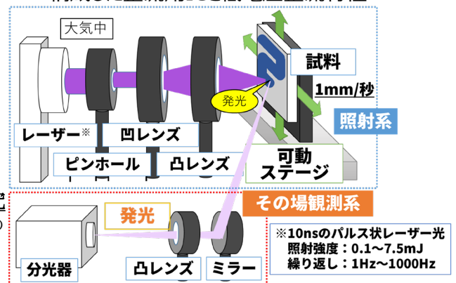
ArFエキシマレーザーを用いた光学系
