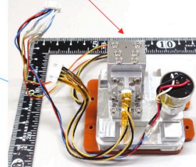
水レジストジェット式 超小型推進器TWEET
