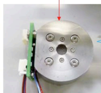
イオン検出用 超小型ファラデーカップ (対気姿勢を計測)
