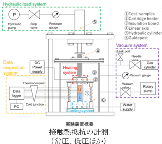
熱伝達係数取得のための実験装置および計測内容
