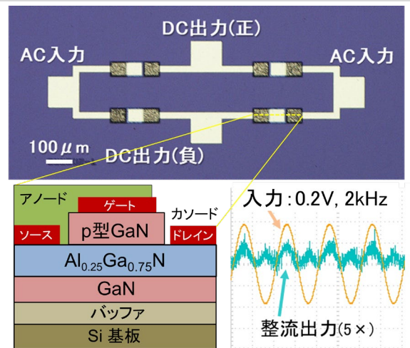
p型GaNゲートヘテロ接合ダイオードで構成した整流用ICと低電圧整流特性
