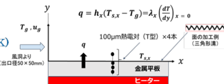
熱伝達係数取得のための実験装置および計測内容
